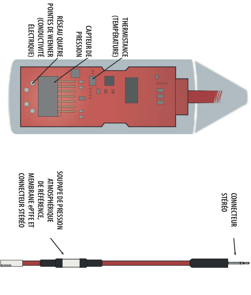
Figure 1 : Schéma des composants du CTD
