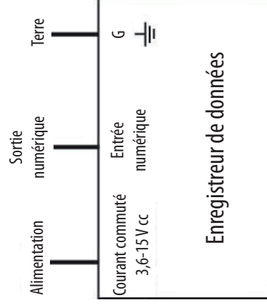
Figure 3 : Schéma de câblage
